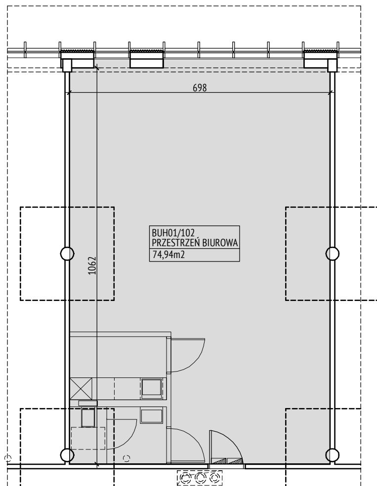
ARANŻACJA POMIESZCZEŃ SANITARNYCH PRZYKŁADOWA
